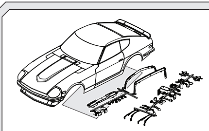
7210 DATSUN 240Z BODY (WB225mm .F0/R3mm) DATSUN 240Z KAROSSERIE (WB225mm .v0mm/h3mm) CARR. DATSUN 240Z (emp 225mm .av0mm/ar3mm) ダットサン240Z ボディー(WB225mm.前0mm/後3mm)
