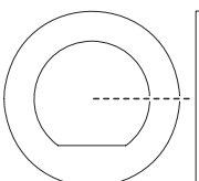
87064 Differential Ring 13.8x21mm D-cut Diff-scheibe 13.8x21mm D-cut Bague différentiel 13.8x21mm forme D デフリング 13.8x21mm Dカット
