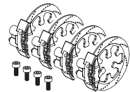
87596 DISK ROTOR / CALIPER SET (GOLD/RED) BREMSSCHEIBE/BREMSSATTEL SET (GOLD/ROT) ENS. DISQUE DE FREINETRIER (OR/ROUGE) ディスクローター/キャリパーセット(レッド/ゴールド)
