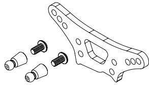
87089 FRONT SHOCK TOWER (WOVEN GRAPHITE/3.0mm) DAEMPFERBRUECKE VORNE (KOHLEFASER/3.0mm) PLATINE AMORTISSEURS AVANT (GRAPHITE TISSE/3mm) リアショックタワー(グラファイト/3.0mm)
