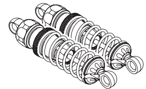
87597 ALUMINUM THREADED SHOCK SET (42-55mm/10mm) ALU GEWINDEDAEMPFER SET (42-55mm/10mm/CR) JEU AMORTISS. ALU. FILETES (42-55mm/10mm) アルミスレッドショックセット(42-55mm/10mm)
