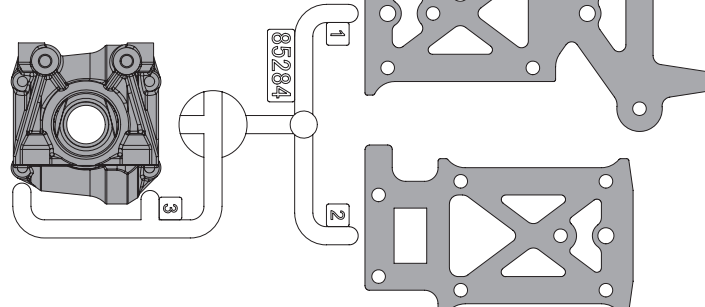
85284 Gear Box B/chassis Spacer Set Getriebe Box B/chassis Spacer Set Ens. boîte engrenages b/piece espacement chassis ギアボックスB/シャーシスペーサーセット
