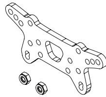
87170 REAR SHOCK TOWER (WOVEN GRAPHITE/3.0mm) DAEMPFERBRUECKE HINTEN (KOHLEFASER/3mm) PLATINE AMORTISSEURS ARRIERE (GRAPHITE TISSE/3mm) リアショックタワー(グラファイト/3.0mm)
