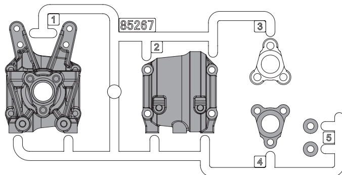
85267 Gear Box Set A Getriebe Box Set A Ens. boîte engrenages A ギアボックスセットA
