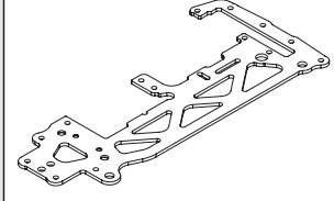
87264 UPPER DECK (WOVEN GRAPHITE/2.0mm) OBERDECK (KOHLEFASER/2.0mm) PLATINE SUPERIEURE (GRAPHITE TISSE) アッパーデッキ(グラファイト/2.0mm)
