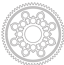
87298 Spur Gear 65tooth (Delrin/48 Pitch) Hauptzahnrad 65 Zähne (Delrin/48DP) Couronne 65D (delrin/48 pitch) スパーギヤ 65T(デルリン/48ピッチ)
